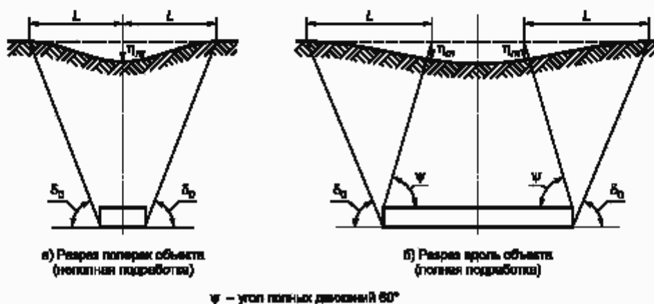
Рисунок С.1 — Основные параметры мульды сдвижения
